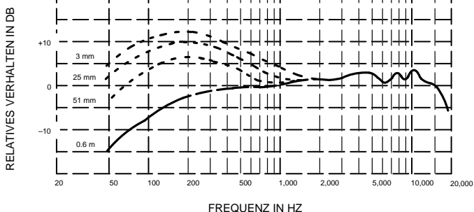
TYPISCHES FREQUENZVERHALTEN ABBILDUNG 2
