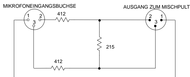
15-DB-DÄMPFUNGSGLIED-SCHALTUNG ABBILDUNG 5
